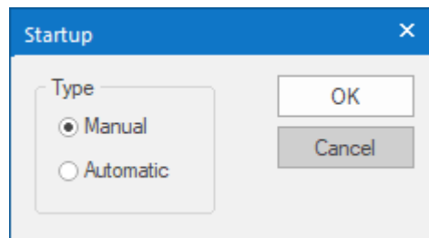
Startup
